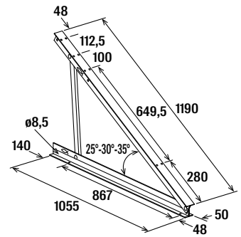
STFN 25°-30°-35°
